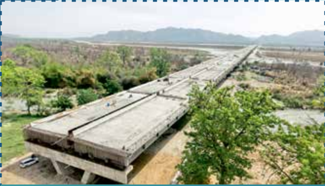
गंगा नदी पर निर्माणाधीन 2.52 किमी लंबा 6 लेन राजमार्ग पुल, हरिद्वार बाईपास परियोजना
